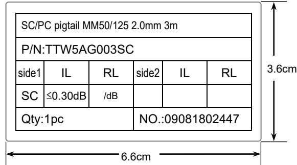
図 1. 貼付ラベルの例 (型番 : TTW5AG003SC 片端 SC/PC コネクタ付き ケーブル長 3m)
