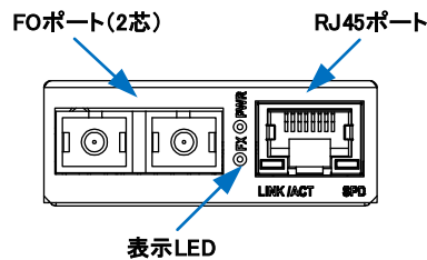
図 1. TMC-302TRSC-F0xx シリーズの装置前面 (表示 LED)
