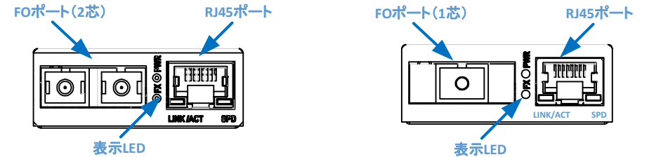
図1. TMC-102TRSxシリーズの前面
