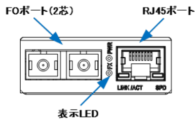
図 1. TMC-102TRSC-F0xx の装置前面 (表示 LED)
