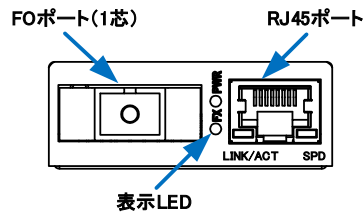
図 1. TMC-102WA/BSC-SMxx シリーズの装置前面 (表示 LED)
