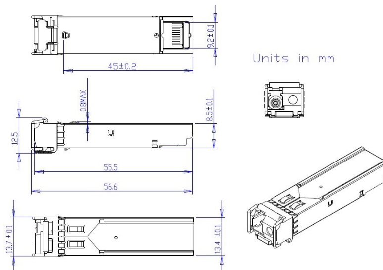
＜LC1 芯タイプ SFP モジュールの外観図 (例)＞
