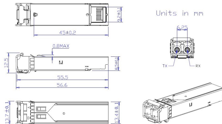
＜LC2 芯タイプ SFP モジュールの外観図 (例)＞
