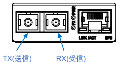
【2 芯タイプ】
