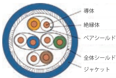
ケーブル断面図
