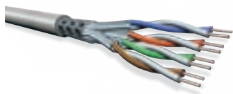
S/FTP 全体編組シールド(S) 各対アルミシールド(FTP)
